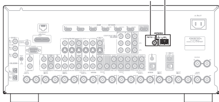
Bornes à poussoir AM ANTENNA Prise FM ANTENNA
