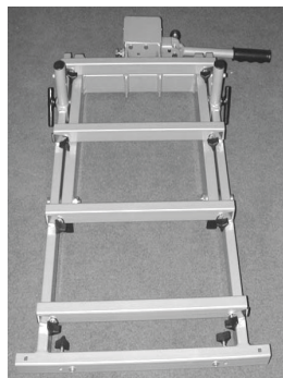
Plateau porteur
