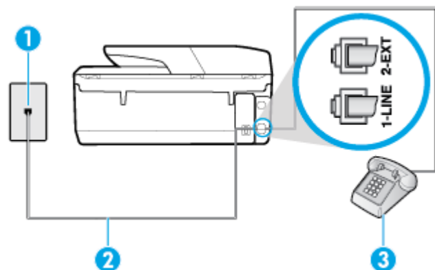
Abbildung 5-4 Rückansicht des Druckers
